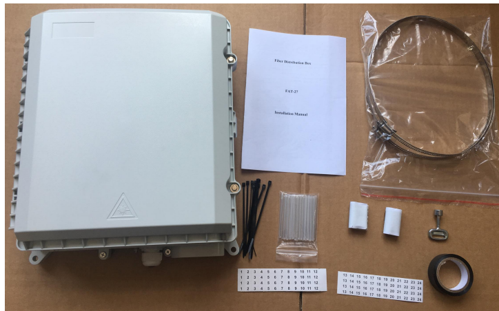
FAT- I -27 型光纤分纤箱选配附件清单
